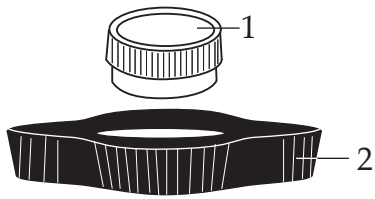
004315 2 Piece Lid
